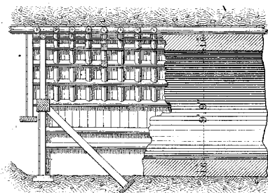
LONGITUDINAL SECTION.
